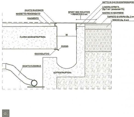
Figura 30 Giunto sismico: a) dettaglio di progetto; b) protezione mediante lamiera striata a scorrimento non impedito.
