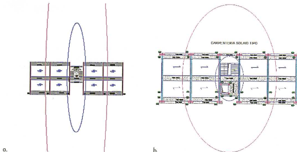
Figura 9 Ellisse centrale d'inerzia degli edifici esistenti a) e di quelli sismicamente rinforzati b).
