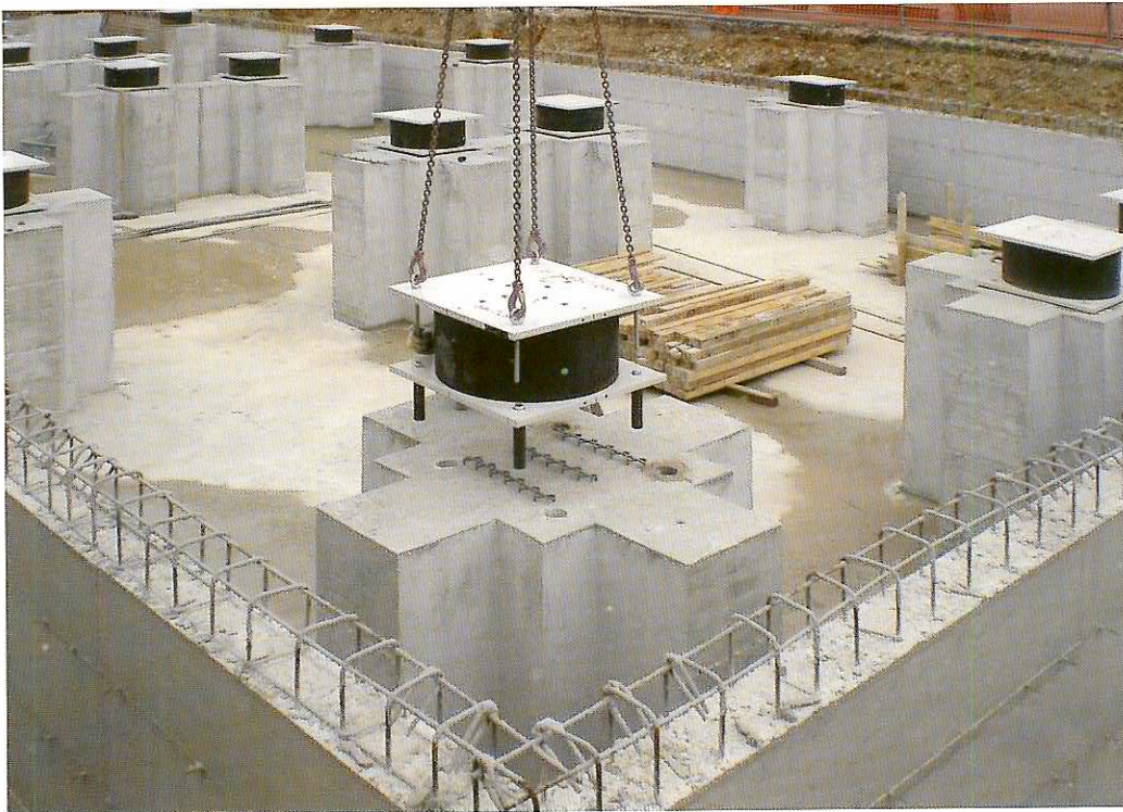
Figura 20 Posa e centraggio degli isolatori.
