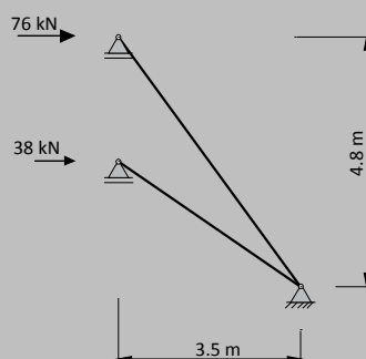
Figura 4.22 Schema di puntello a fasci convergenti.
