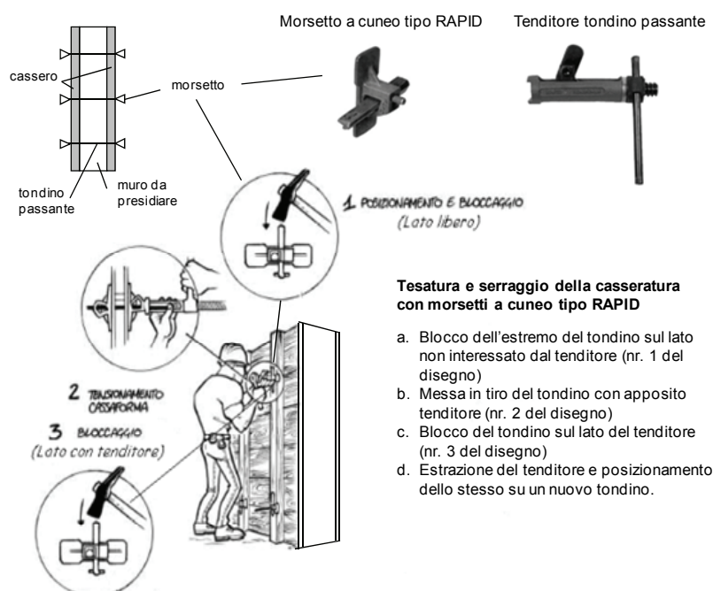
Figura 4.89 Descrizione sintetica delle fasi esecutive dell'incamiciatura di pareti.
