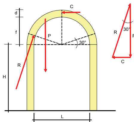
Figura 4.60 Schema di calcolo delle centine.
