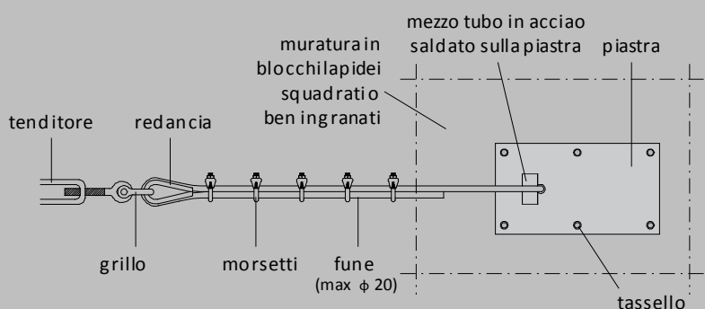
Figura 4.79 Fune passante in foro: particolare della deviazione del cavo attraverso un foro nella muratura e relativa piastra di rinforzo.
