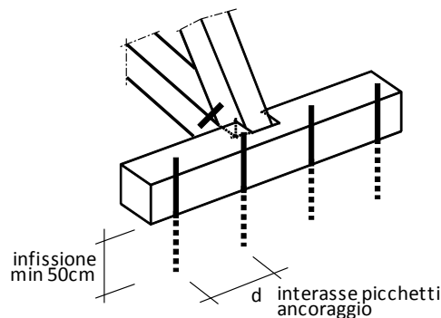
Figura 4.19 Particolare dell'ancoraggio a terra delle puntellature su base di appoggio. I picchetti devono essere infissi sul terreno per una profondità di almeno 50 cm e posti ad interasse d come indicato nel Vademecum STOP nella scheda PR.
