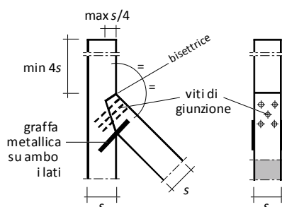
Nodo superiore ritto-puntone
