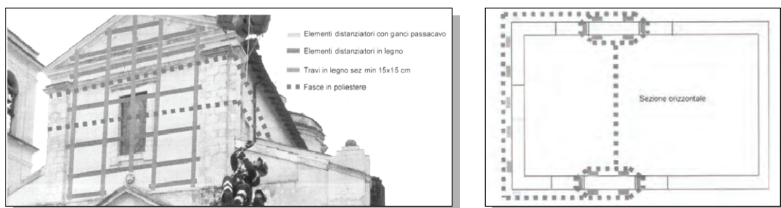
Graticcio ligneo tirantato con fasce di poliestere nella parte alta della facciata (Archivio NCP).
