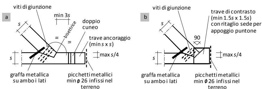
Figura 4.18 Caratteristiche geometriche dei giunti e lunghezza minima del tallone per giunti sul ritto e sulla base.
