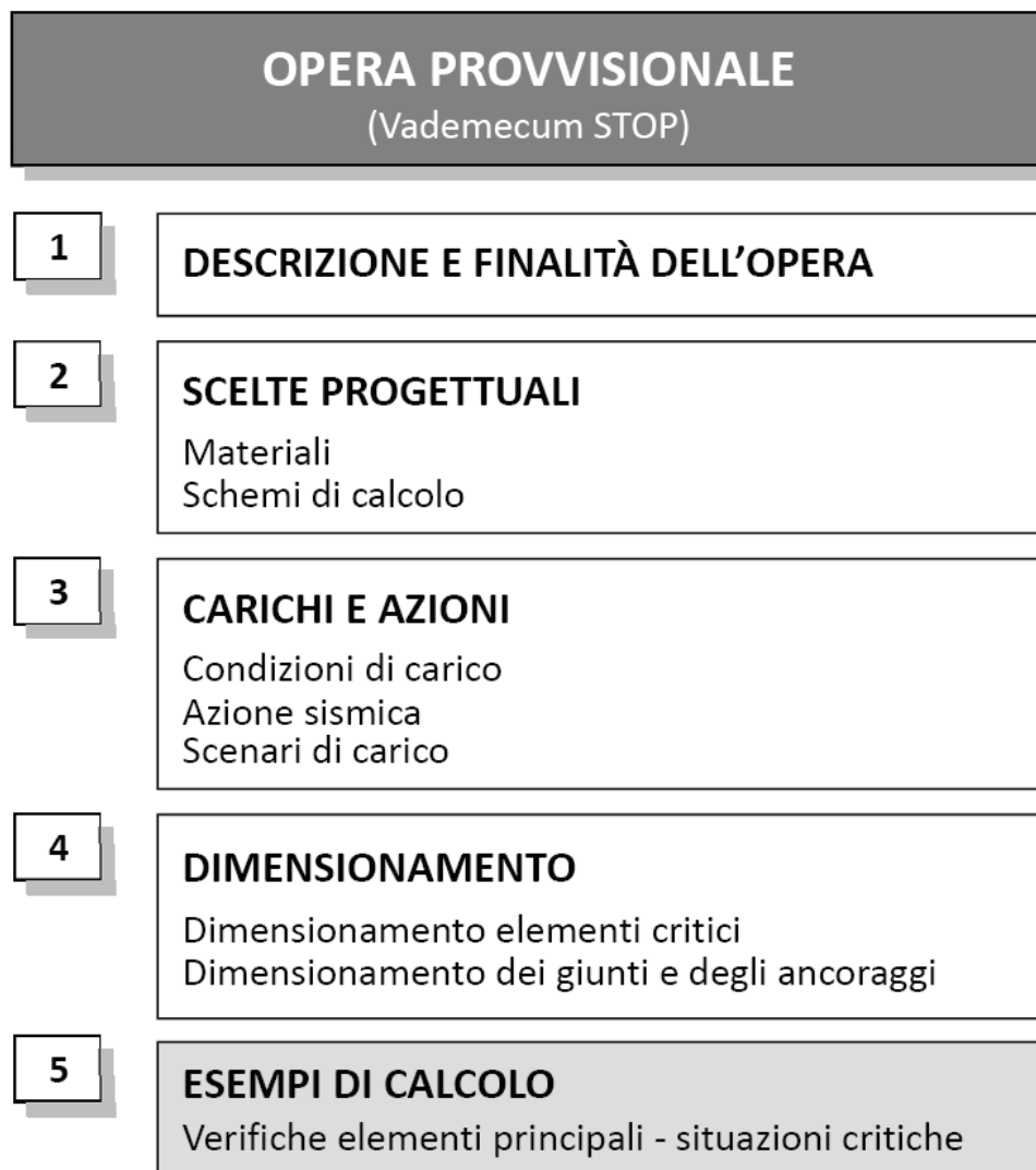
Figura 4.1 Struttura logica utilizzata per illustrare i criteri e le ipotesi alla base del dimensionamento delle opere provvisionali del Vademecum STOP
